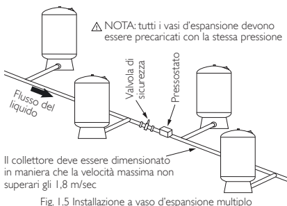
Fig. I.5 Installazione a vaso d'espansione multiplo
