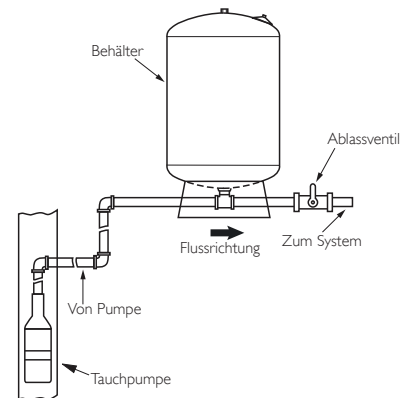
Abb. I.4-3 Mit Tauchpumpe
