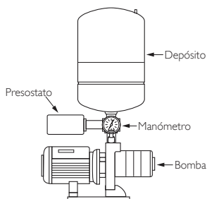
Fig. I.4-5 Bomba cebadora con depósito en línea
