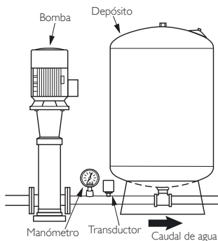
Fig. I.4-6 Bomba cebadora con depósito
