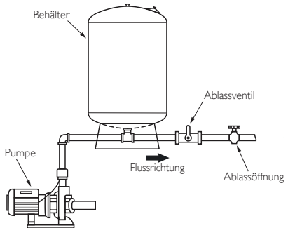
Abb. I.4-2 Mit wendelbarer Vielzweck-Jetpumpe
