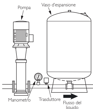
Fig. I.4-6 Installazione su gruppo aumento pressione con vaso
