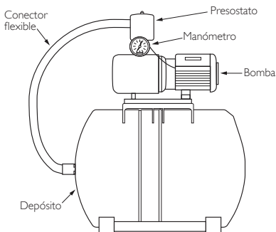
Fig. I.4-4 Bomba cebadora c/ depósito horizontal
