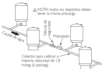
Fig. I.5 Instalación multidepósitos
