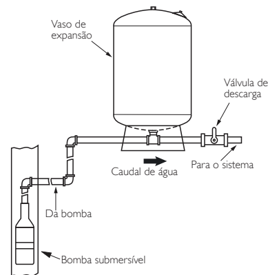
Fig. 1.4-3 Com bomba submersível
