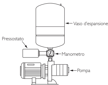
Fig. I.4-5 Installazione su gruppo aumento pressione con vaso Inline
