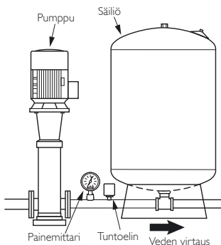
Kuva 1.4-6 Paineenkorotuspumppu
