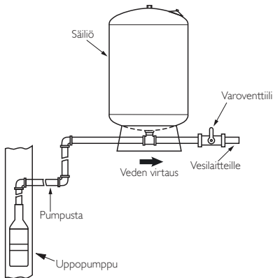
Kuva 1.4-3 Asennus uoppopumpun kanssa
