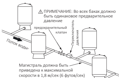
Рис. 1.5 Установка нескольких баков
